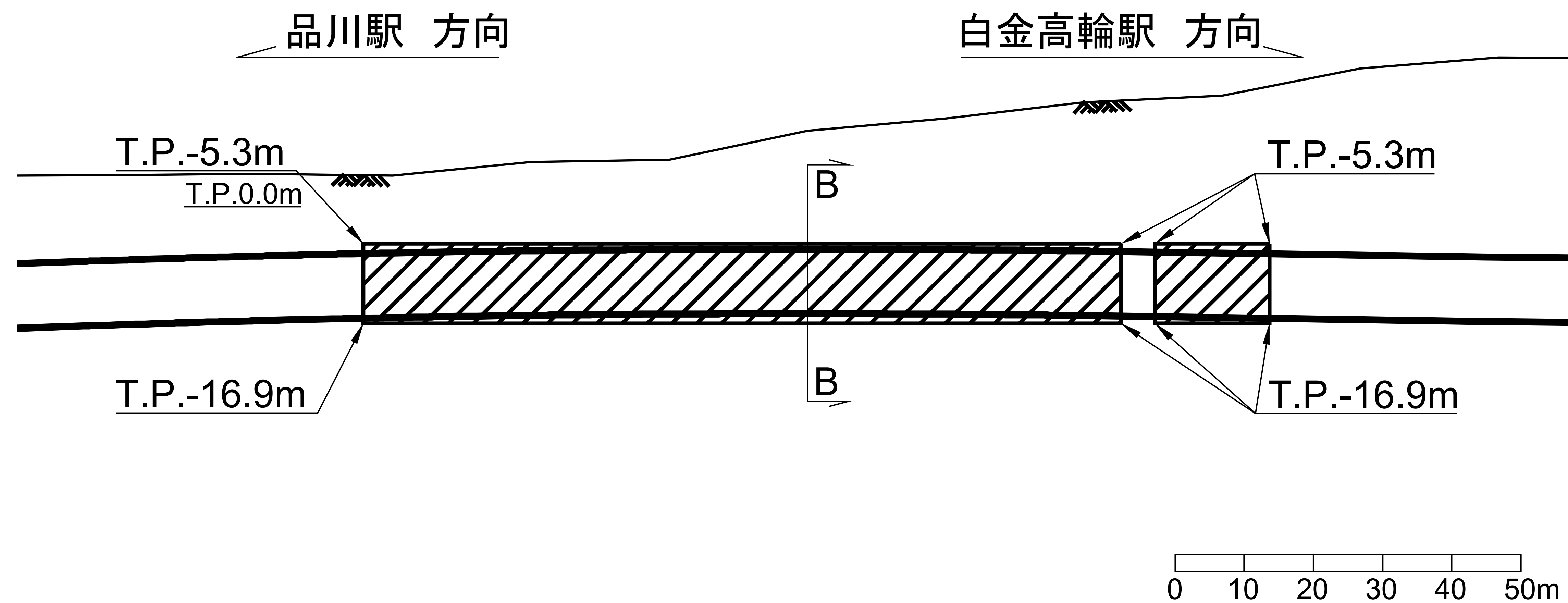
A-A断面図
