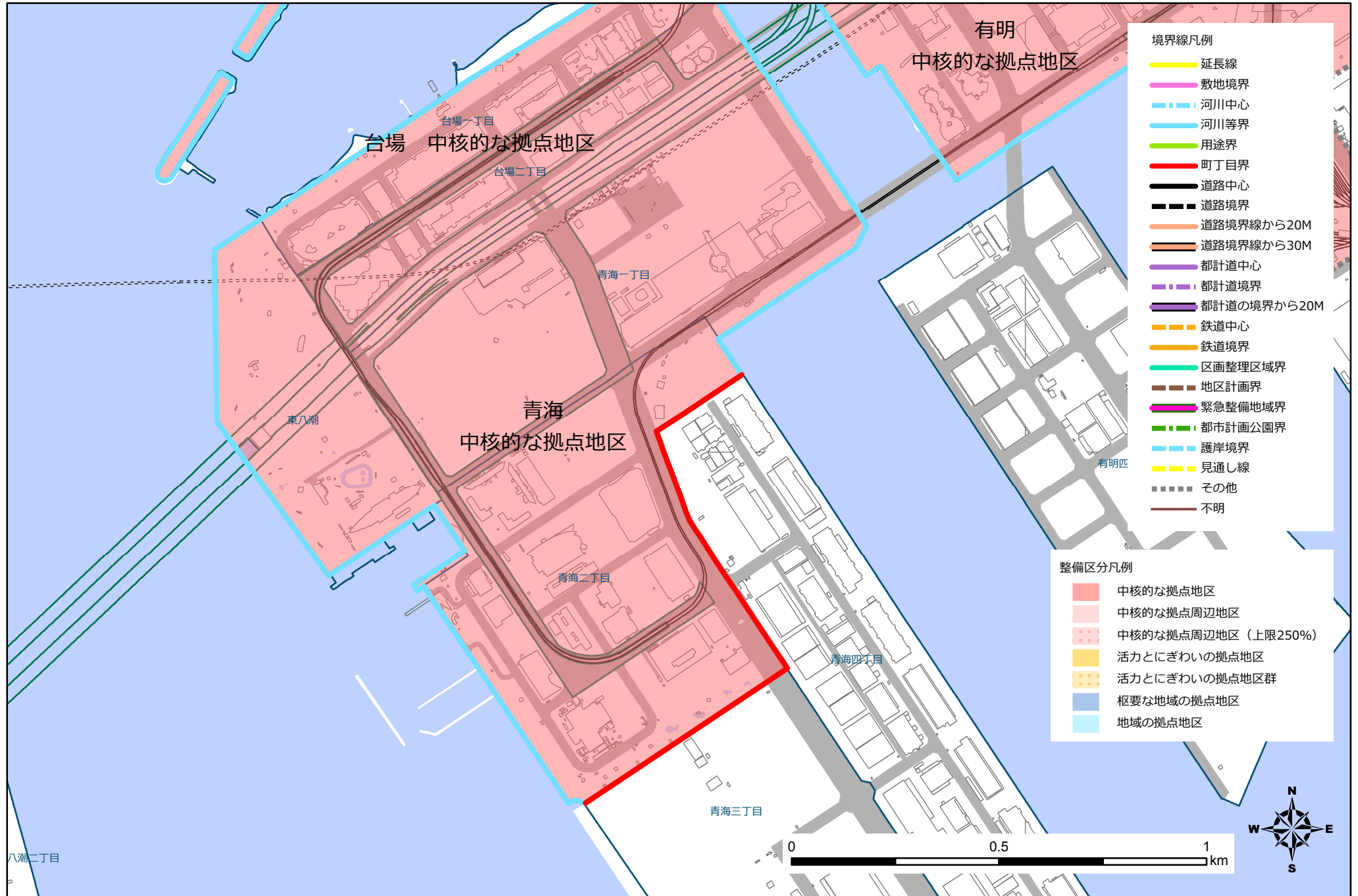
図C-21 青海 中核的な拠点地区範囲図
