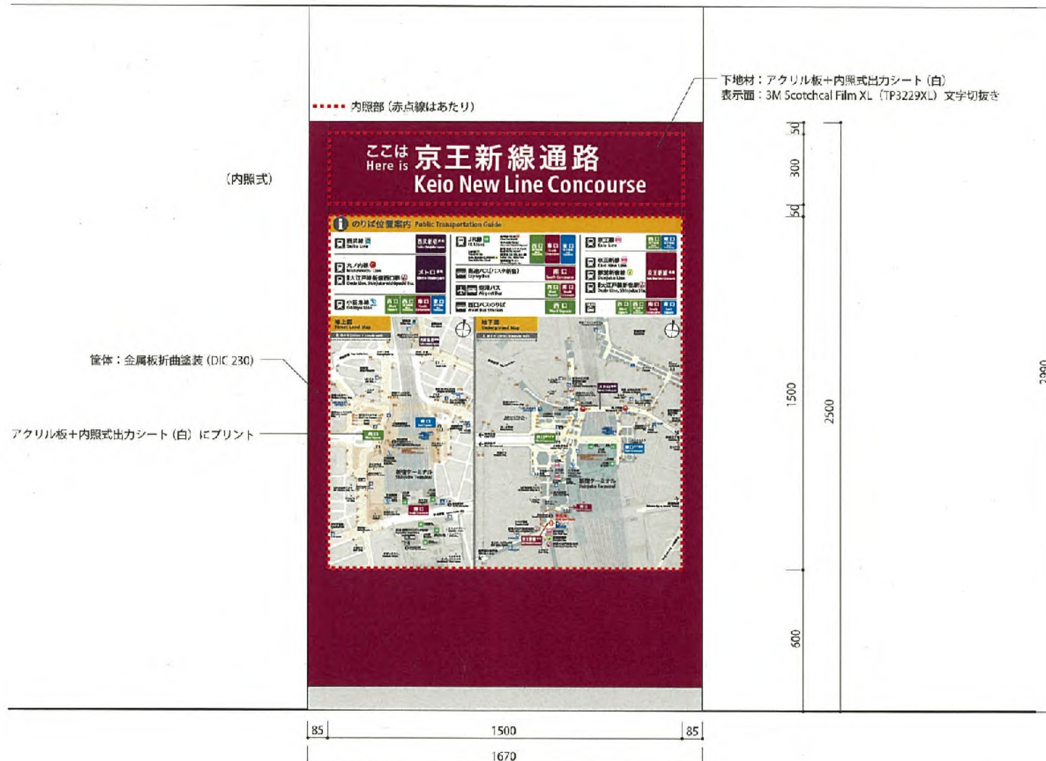
K3-図01 器具外形寸法H2500×W1670 (タイトル和文文字高110)
