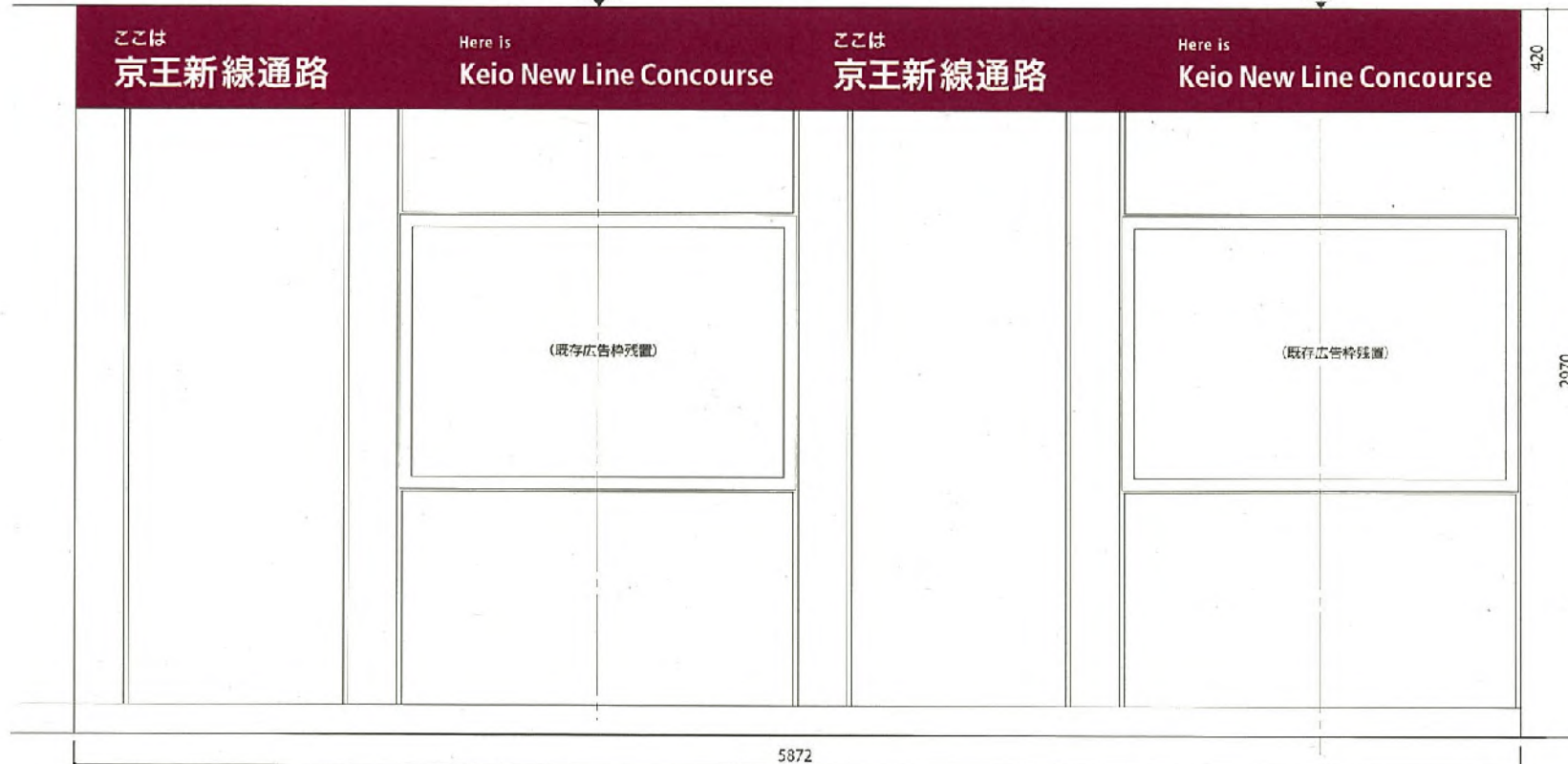
K③-27 器具外形寸法H420×W5872 (和文文字高130)
