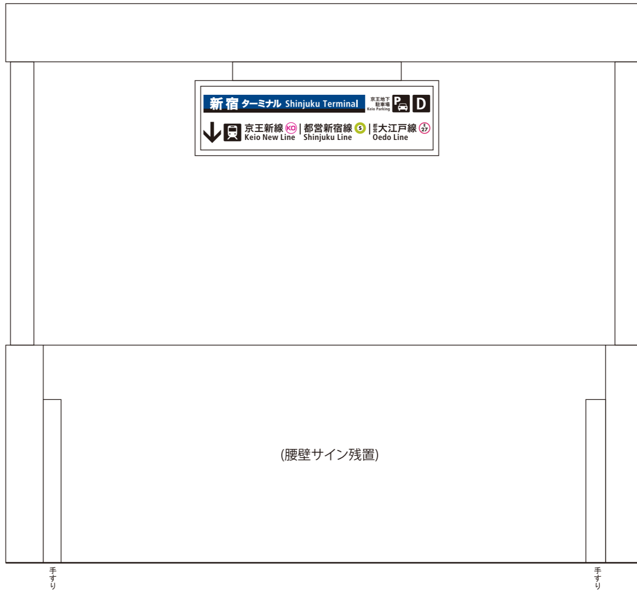
西-1003<両面>オモテウラ共 表示面寸法H340×W1240 (和文文字高64,47,23.4)
