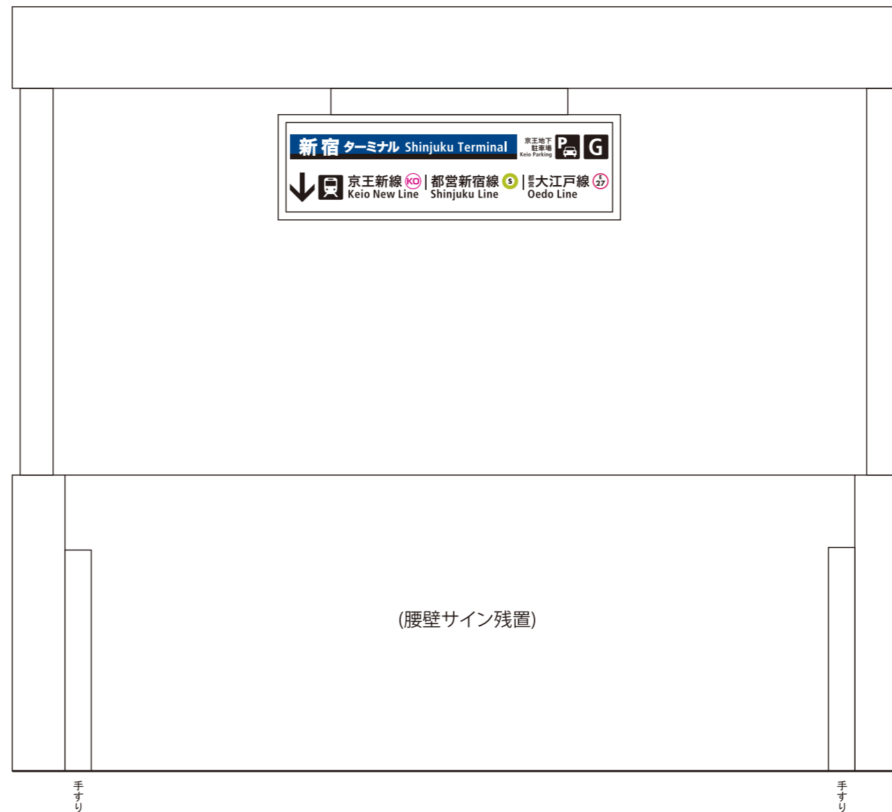
西-1006<両面>オモテウラ共 表示面寸法H340×W1240 (和文文字高64,47,23.4)
