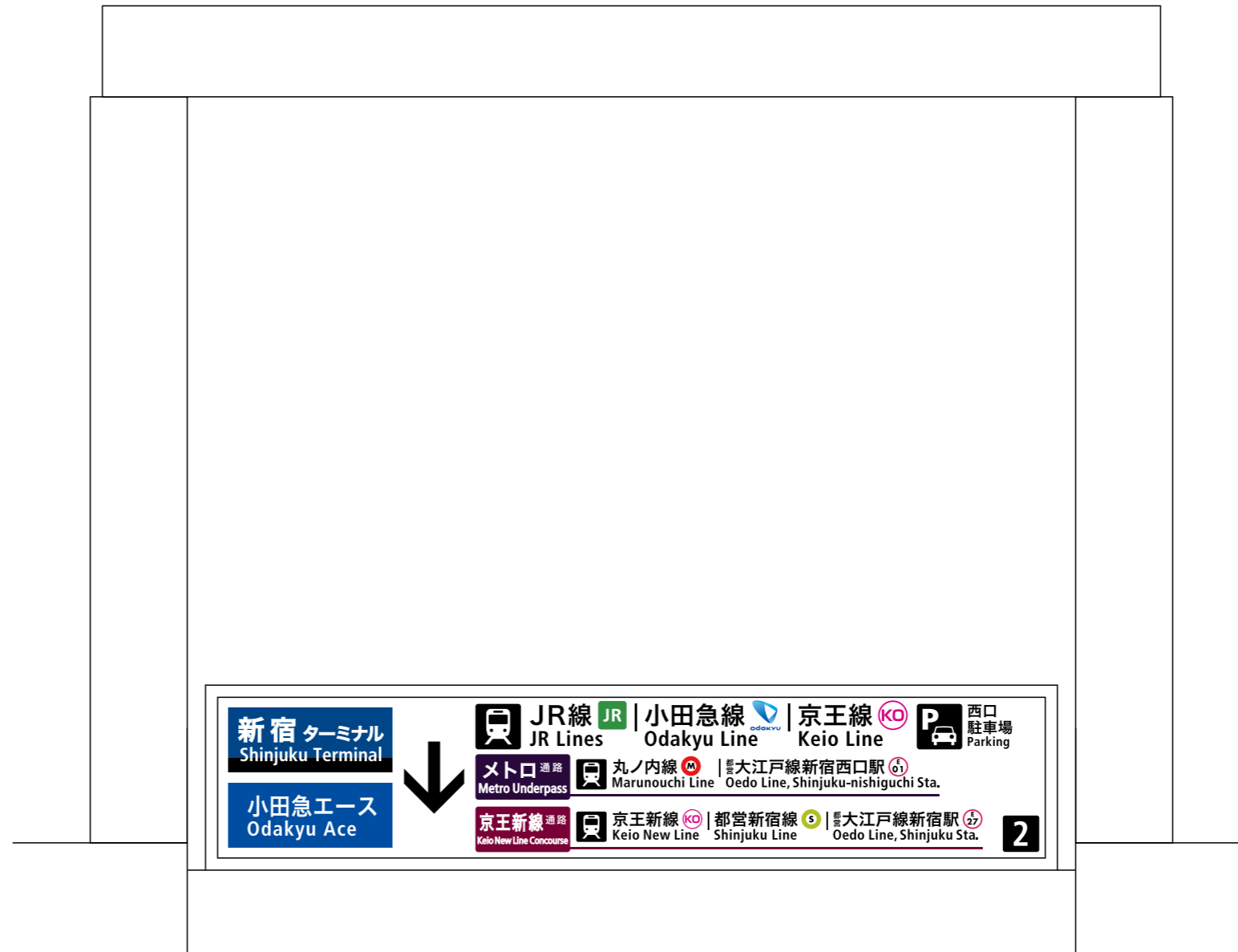
西-4002<片面> 表示面寸法H530×W2730 (和文文字高81,75,72,50,45.5)
