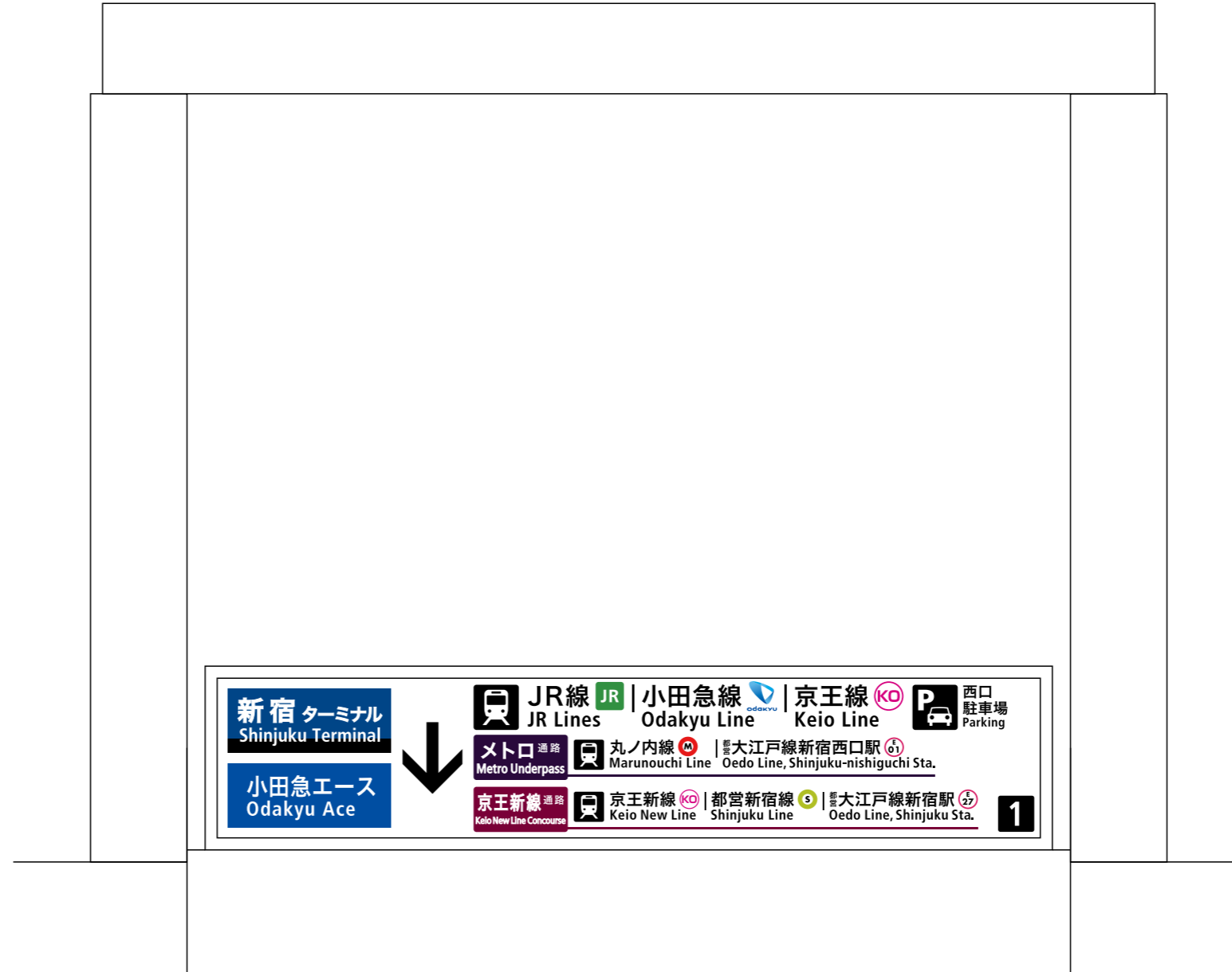
西-4001<片面> 表示面寸法H530×W2730 (和文文字高81,75,72,50,45.5)
