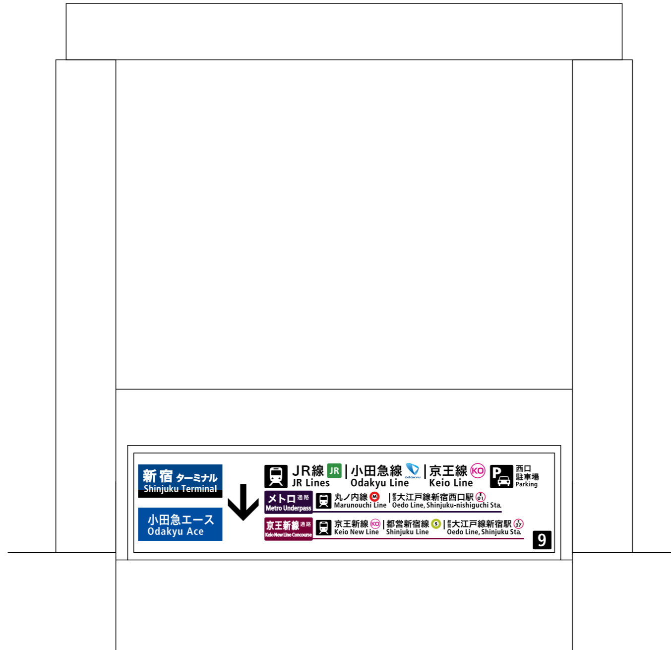
西-4008<片面> 表示面寸法H530×W2230 (和文文字高79.5,66.9,62,41.3,37.6)
