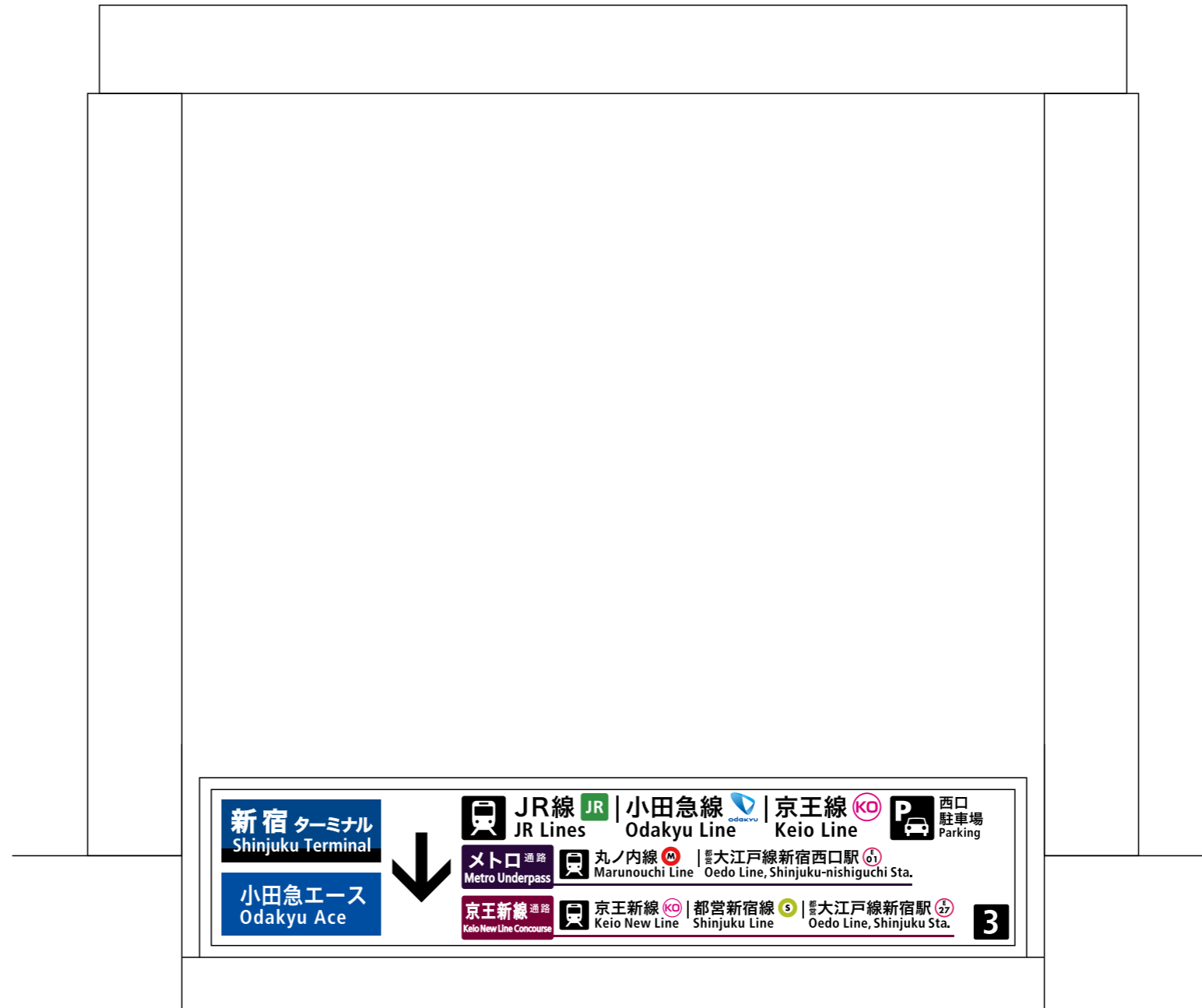
西-4003<片面> 表示面寸法H530×W2730 (和文文字高81,75,72,50,45.5)
