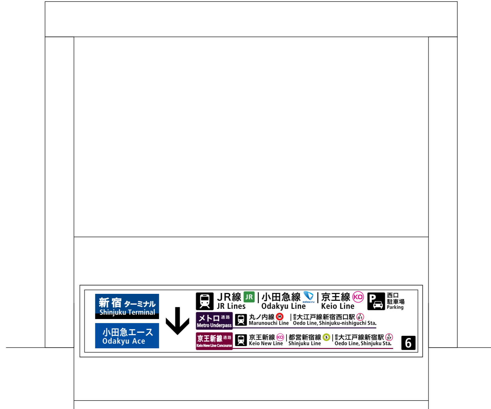
西-4006<片面> 表示面寸法H530×W2830 (和文文字高81,75,72,50,45.5)
