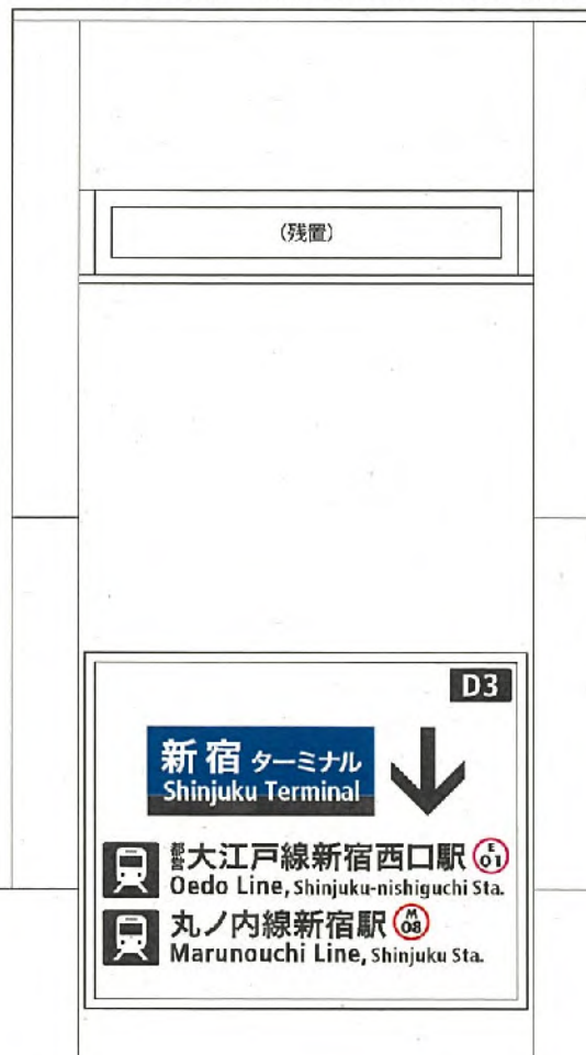
西-5004<片面> 表示面寸法H1195×W1495 (和文文字高130,100)
