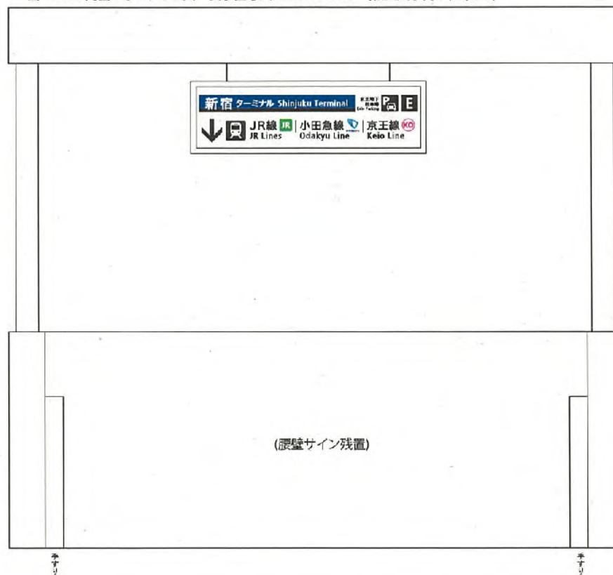
西-1004<両面>オモテウラ共 表示面寸法H340×W1240 (和文文字高64,55,23.4)
