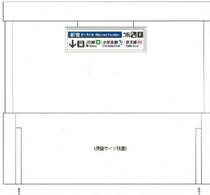
西-1005<両面>オモテウラ共 表示面寸法H340×W1240 (和文文字高64,55,23.4)
