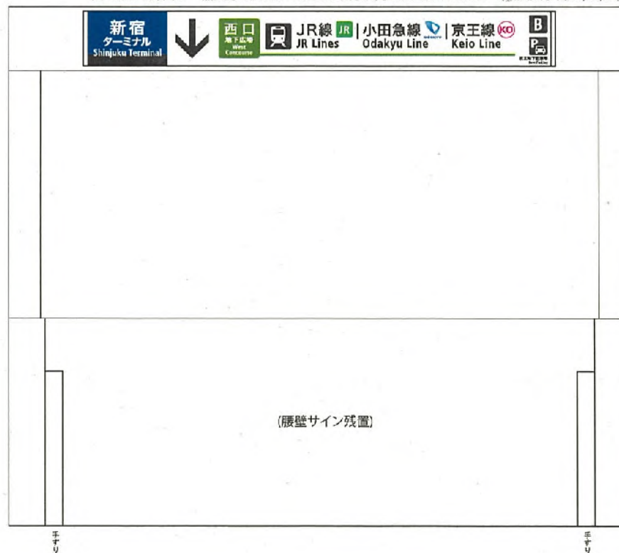
西-1001<片面> 器具寸法H300×W2580 表示面寸法H300×W2530 (和文文字高80,72,20)
