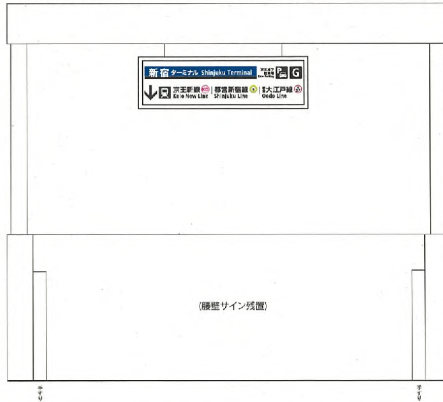
西-1006<両面>オモテウラ共 表示面寸法H340×W1240 (和文字高64,47,23.4)
