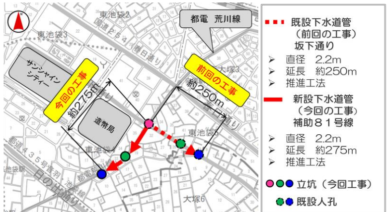
▶ 幹線下水道整備の工事概要
