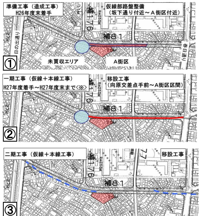
▲ 軌道工事の予定
