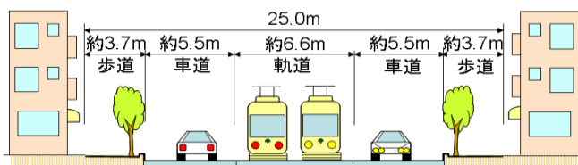
▲ 道路全体の整備イメージ
