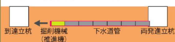
下水道工事（推進工法）のイメージ図
