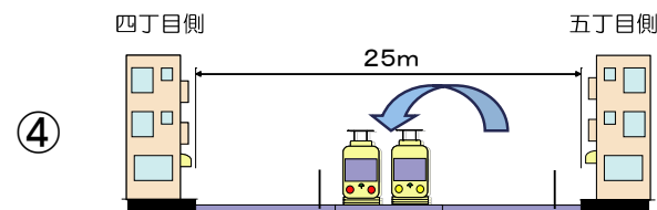
本線への切替工事(夜間)
